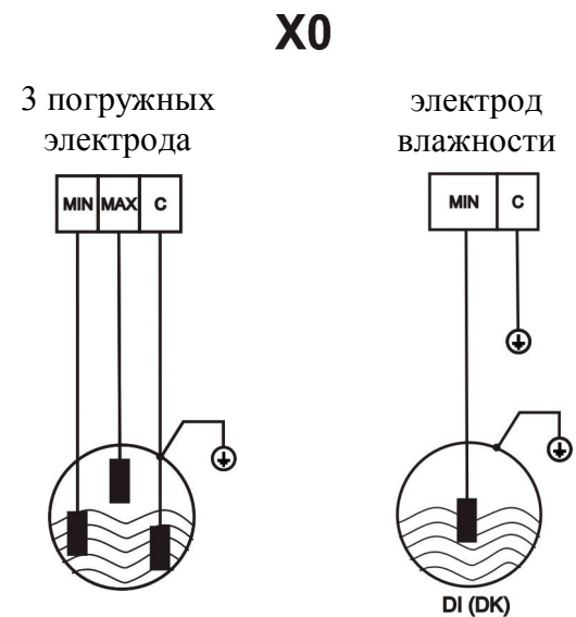
Рис. 3 Схема подсоединения сетевых контактов и клеммных колодок
